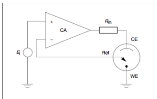
Figura 9: Schema elettrico dell'amplificatore operativo
